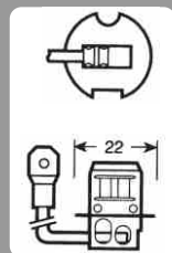
Cód. 80720 112 11 H3, 12V 55W PLASMA XENON Zócalo: PK 22s Uso: faros auxiliares
