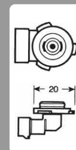
Cód. 80720 116 3 Hb3 9005, 12V 65W Zócalo: P 20d Uso: alta y baja
