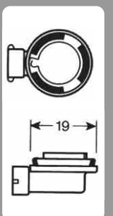
Cód. 80720 116 4 H11, 12V 55W Zócalo: PGJ 19 Uso: alta o baja
