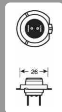
Cód. 80720 114 11 H7, 12V 55W PLASMA XENON Zócalo: PX 26d Uso: alta y baja
