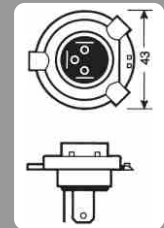
Cód. 80720 110 17 H4, 12V 60/55W PLASMA XENON Zócalo: P 43t Uso: alta y baja
